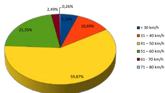
Avenue Jean Moulin sens descendant zone 50
